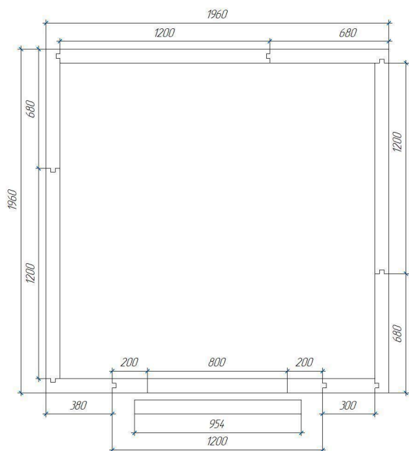
Схема построения стен (вид сверху) (вид сверху).
