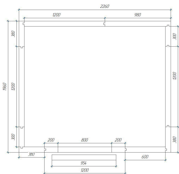
Схема построения стен (вид сверху) (вид сверху).
