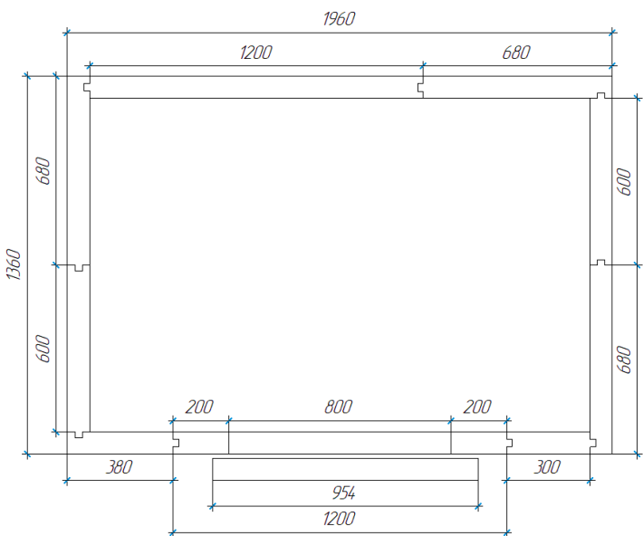
Схема построения стен (вид сверху) (вид сверху).
