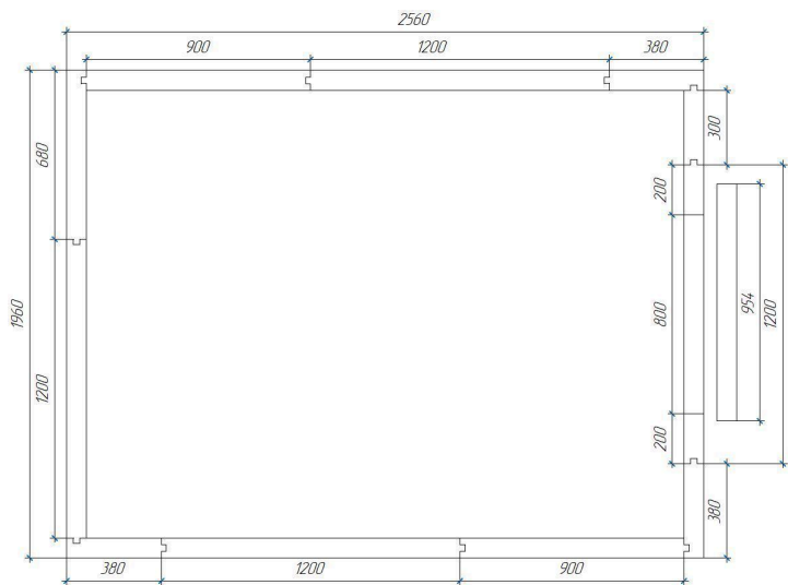
Схема построения стен (вид сверху) (вид сверху).
