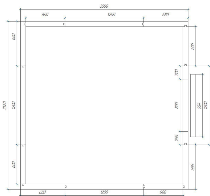
Схема построения стен (вид сверху) (вид сверху).
