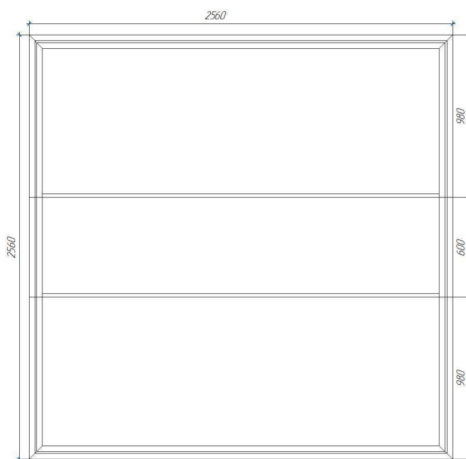
Схема построения пола, потолка
